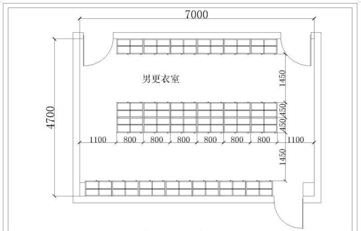
女更衣室衣柜平面图
